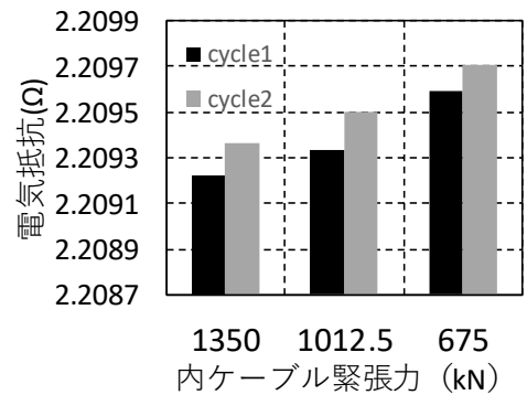
図-4 電気抵抗の平均値 (温度補正後)
