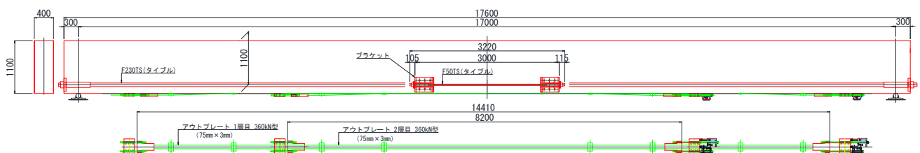
図-1 試験体
