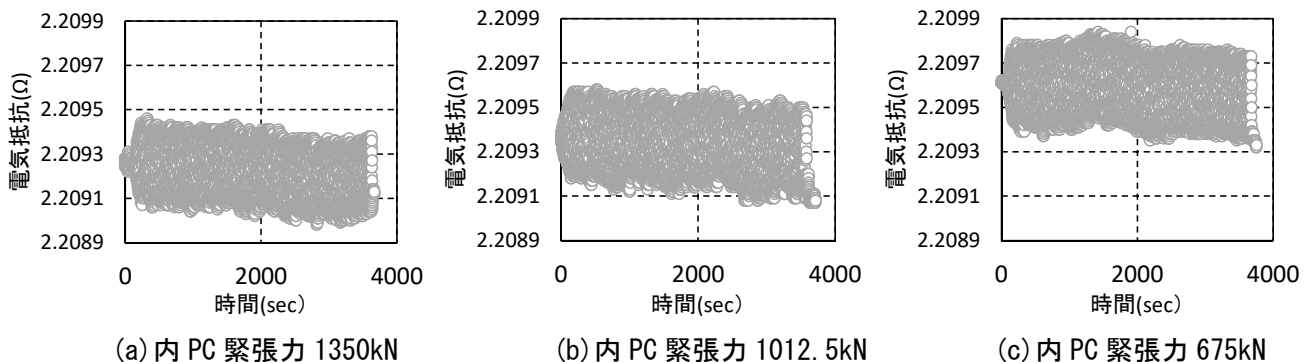
図-3 CFRP1 層目 繰返し载荷時の電気抵抗 (温度補正後)
