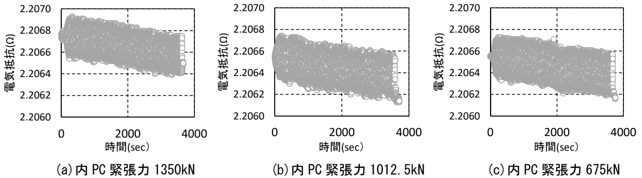
図-2 CFRP1 層目 繰返し载荷時の電気抵抗 (温度補正前)
